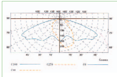
Ένταση [cd/1000lm] Intensity[cd/1000lm] Πολικό διάγραμμα Coral Polar diagram Coral
